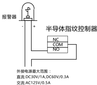
报警输出接线示意图
