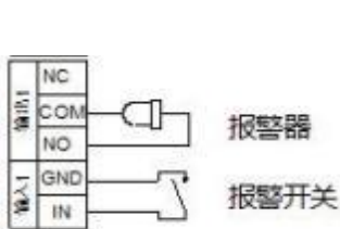
图一 有源接法
